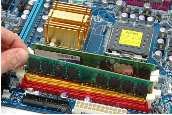
Şekil 18 Anakarta takılı RAM
