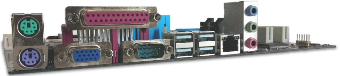
Şekil 15 Anakart üzerindeki bağlantı noktaları
